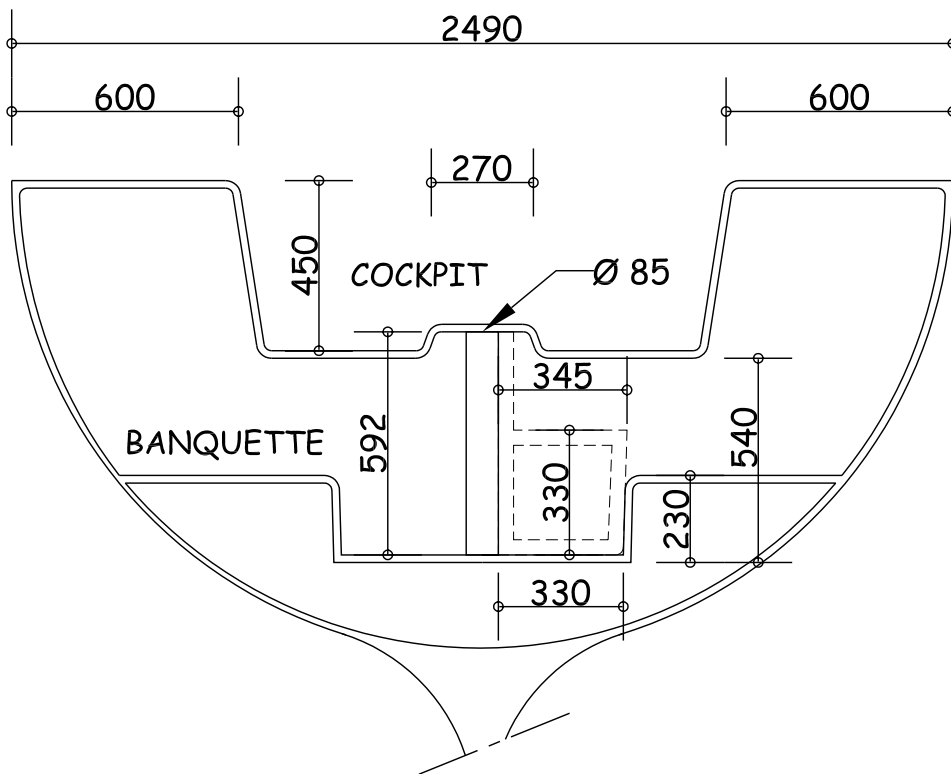
COUPE VUE VERS LA POUPE
